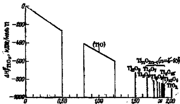
Рис. 3.33. Зависимость стандартной энтальпии образования оксидов титана от кислородного индекса.
