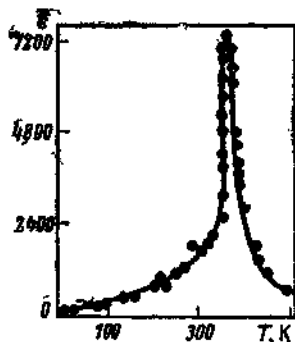
Рис. 3.8. Зависимость диэлектрической проницаемости титаната бария от температуры.
