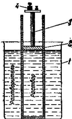
Рис. 2.27. Схема опыта, поясняющего осмотическое давление: 1—сосуд с растворителем; 2—сосуд с раствором; 3—поршень; 4—груз.
