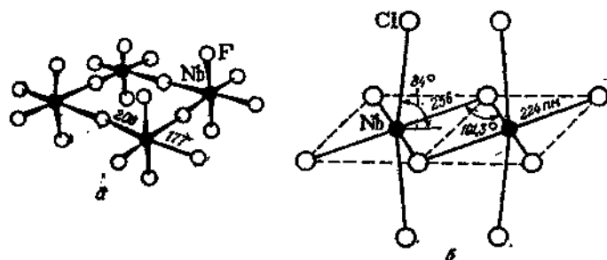
Рис. 3.107. Структура полимеров, образующих кристаллы NbF_5 :
