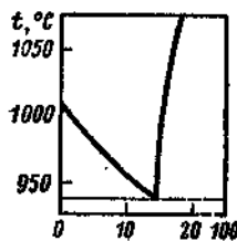
Рис. 3.11. Фрагмент диаграммы состояния системы \text{Na}_3\text{AlF}_6 — \text{Al}_2\text{O}_3 .
