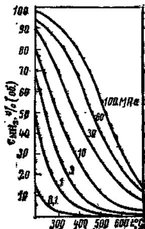
Рис. 3.44. Зависимость равновесного выхода аммиака от температуры и давления.
