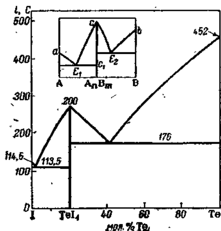
Рис. 2.36. Диаграмма состояния системы из веществ, образующих устойчивое химическое соединение A_nB_m .
