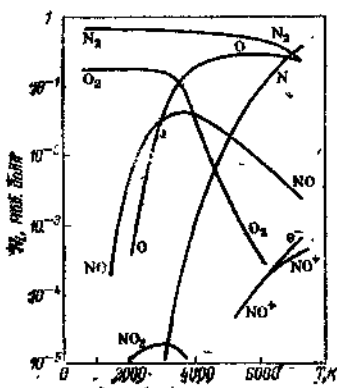
Рис. 2.12. Зависимость равновесного состава воздуха (смесь азота и кислорода) от температуры T .
