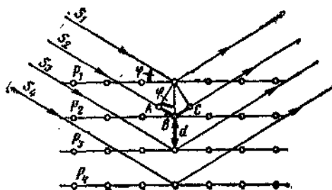
Рис. 1.77. Схема, поясняющая вывод уравнения Брегга — Вульфа.
