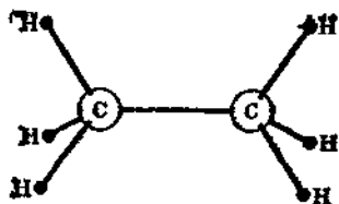
Рис. 142. Строение молекулы C_2H_6 .
