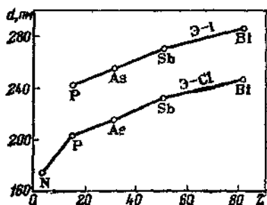
Рис. 1.15. Зависимость межатомных расстояний d-N-I и d-N-Cl от порядкового номера элемента.
