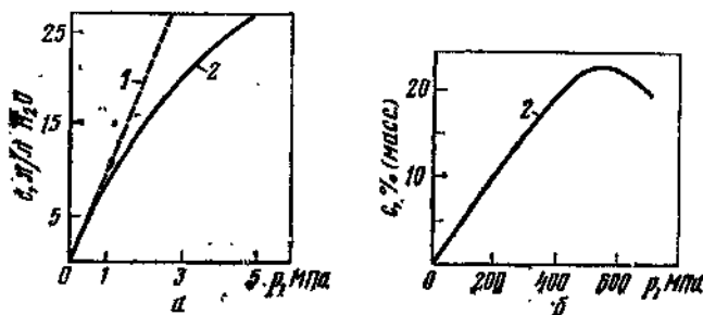
Рис. 2.22. Зависимость растворимости \text{CO}_2 в воде при 15^{\circ}\text{C} (а) и \text{N}_2 в жидком диоксиде серы при 25^{\circ}\text{C} (б) от давления; 1 — по закону Генри; 2 — экспериментальные данные.
