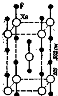
Рис. 3.88. Кристаллическая решетка \text{XeF}_2 .
