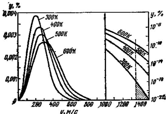
Рис. 2.14. Кривые распределения скоростей молекул N_2O_5(g) при различных температурах y — содержание молекул, скорость которых лежит в пределах между u^* и u + 0,01 м/с.
