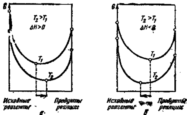
Рис. 2.11. Влияние температуры на химическое равновесие при p = \text{const} : а — эндотермическая реакция; б — экзотермическая реакция. По оси абсцисс отложен состав смеси.
