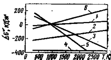
Рис. 2.9. Зависимость \Delta G^\circ от температуры T для реакций:
