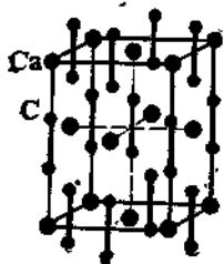
Рис. 3.6. Кристаллическая решетка карбида кальция.
