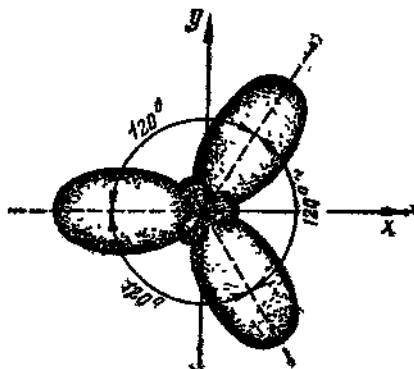
Рис. 138. Пространственное расположение гибридных электронных облаков атома углерода.
