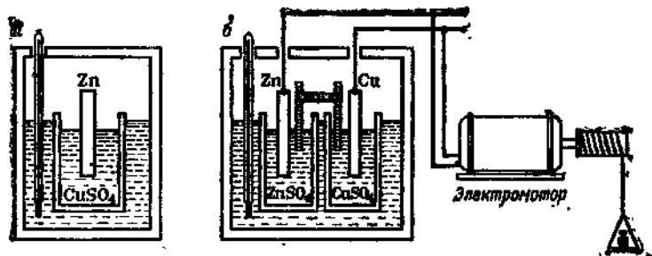
Рис. 2.10. Варианты проведения реакции \text{Zn (к)} + \text{CuSO}_4 (\text{р}) \rightarrow \text{Cu (к)} + \text{ZnSO}_4 (\text{р}) при 25^\circ\text{C} и 101 \text{ кПа} ;
