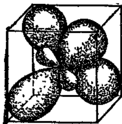
Рис. 138. Пространственное расположение гибридных электронных облаков атома углерода.
