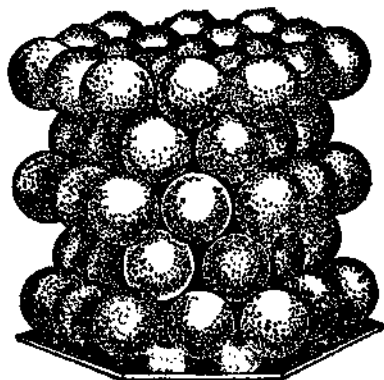
Рис. 1.82. Плотнейшие упаковки шаров:
