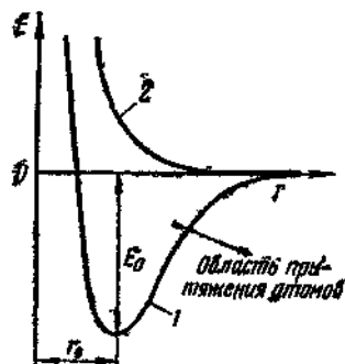
Рис. 130. Кривая энергии устойчивой молекулы (1) и системы из двух атомов, между которыми не образуется химическая связь (2).
