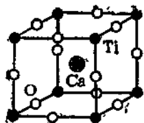
Рис. 3.103. Структура перовскита.
