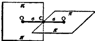
Рис. 145. Схема, показывающая образование химических связей в молекуле CO_2 .
