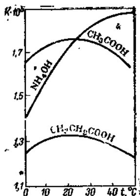
Рис. 2.30. Зависимость константы диссоциации некоторых слабых электролитов в водных растворах от температуры.
