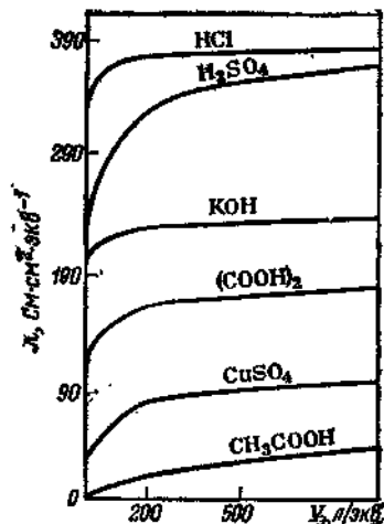
Рис. 2.28. Зависимость эквивалентной электропроводности от разбавления для водных растворов некоторых электролитов при 25 °C.
