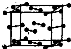
Рис. 3.83. Кристаллическая решетка льда.
