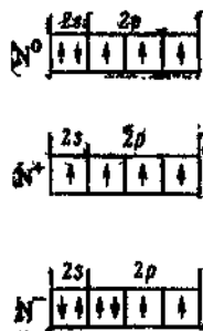
Рис. 3.42. Распределение электронов по квантовым ячейкам в атоме азота и образованных из него ионах.
