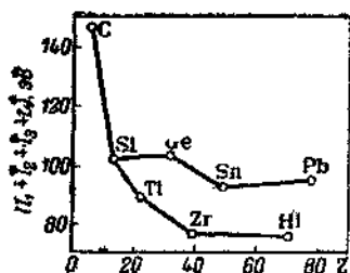
Рис. 117. Зависимость суммы первых четырех энергий ионизации атомов элементов IV группы от порядкового номера элемента.
