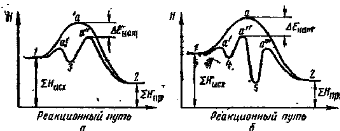
Рис. 2.17. Схема протекания процесса при гомогенном катализе (кривая 1— \alpha' —3— \alpha'' —2) и гетерогенном катализе (кривая 1— \alpha' —4— \alpha'' —5— \alpha''' —2).
