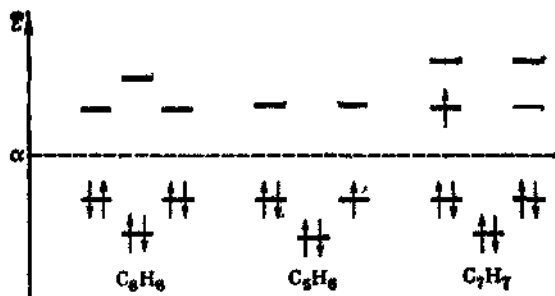
Рис. 1.54. Уровни энергии \pi -электронов в циклических молекулах C_6H_6 , C_5H_5 , C_7H_7 .
