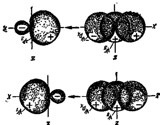
Рис. 1.37 Построение sp -гибридных орбиталей из s - и p -орбиталей.
