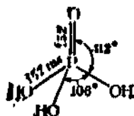
Рис. 3.57. Строение молекулы H_3PO_4 .
