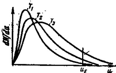
Рис. 2.15. Кривые распределения молекул по их кинетической энергии при разных температурах ( T_3 > T_2 > T_1 ).
