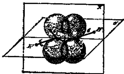
Рис. 1.43. Схема, показывающая образование химических связей в молекуле C_2H_4 .
