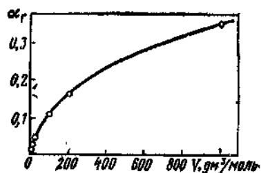
Рис. 2.32. Зависимость степеней гидролиза \text{Na}_2\text{CO}_3 от разбавления при 20 °C.
