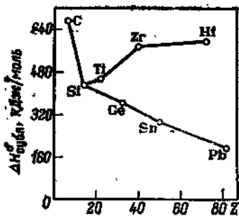
Рис. 3.01. Зависимость стандартной энтальпии сублимации элементарных веществ IV группы от порядкового номера элемента.
