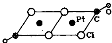
Рис. 3.138. Структура [\text{PtCl}_2(\text{CO})]_2 .
