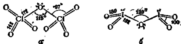
Рис. 3.80. Строение молекул \text{Cl}_2\text{O}_7 (а) и \text{I}_2\text{O}_5 (б).
