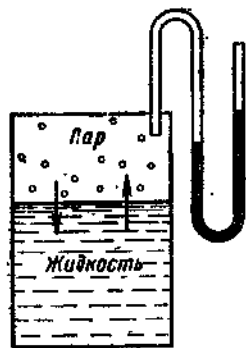
Рис. 2.25. Схема измерения давления насыщенного пара.
