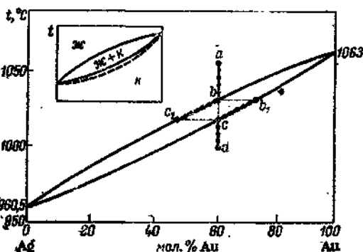
Рис. 2.38. Диаграмма состояния системы из веществ, образующих твердые растворы:
