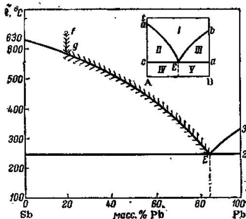
Рис. 2.35. Диаграмма состояния системы из веществ, образующих эвтектическую смесь.
