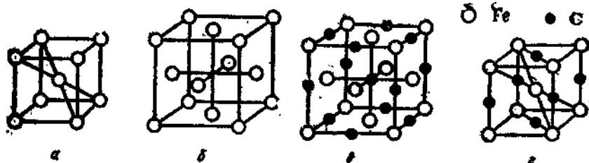
Рис. 3.123. Кристаллические структуры \alpha -Fe (а), \gamma -Fe (б), аустенита (в), мартенсита (г).
