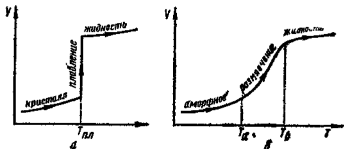
Рис. 1.92. Изменение объема при нагревании кристаллических (а) и аморфных (б) веществ.
