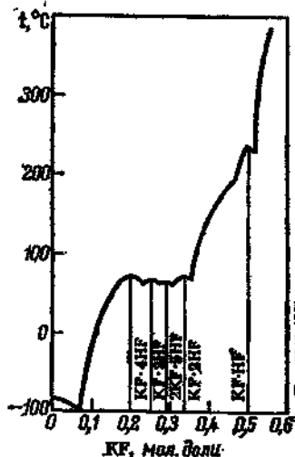
Рис. 3.78. Фрагмент диаграммы состояния системы HF—KF.
