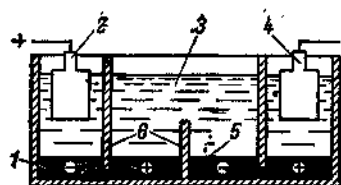
Рис. 3.149. Схема электролизера для очистки индия амальгамным методом:
