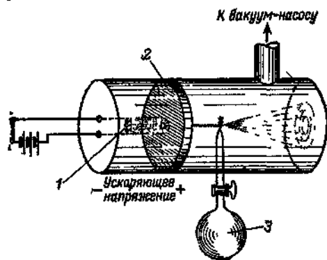
Рис. 1.24. Принципиальная схема электронографа:
