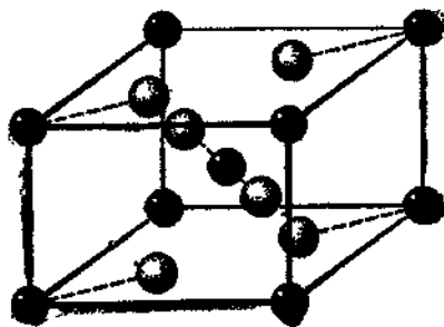
Рис. 1.89. Структура рутила. Светлые шары — атомы O , темные — атомы Ti .
