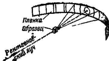
Рис. 1.79. Схема регистрации дебаграммы.
