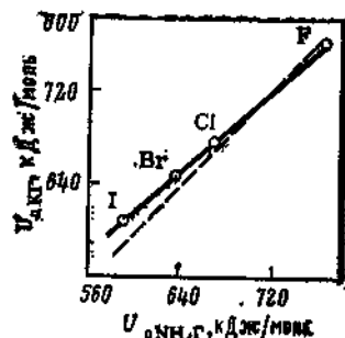
Рис. 3.46. Взаимосвязь между энергиями кристаллической решетки U_0 галогенидов аммония и калия. Пунктир отвечает равенству значений U_0 .
