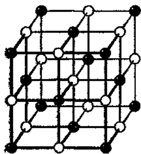
Рис. 1.84. Кристаллическая решетка хлорида натрия.
