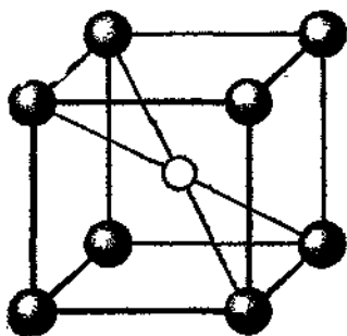
Рис. 1.83. Кристаллическая решетка хлорида цезия.
