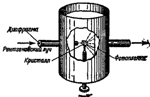
Рис. 178. Камера для получения рентгенограмм по методу вращения кристалла.
