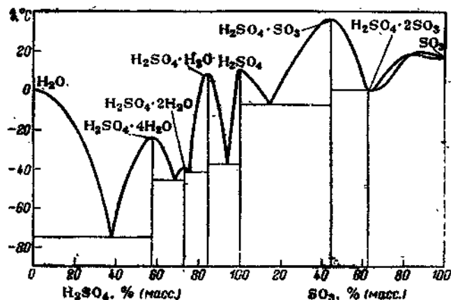
Рис. 3.69. Совмещенные диаграммы состояния систем \text{H}_2\text{O}-\text{H}_2\text{SO}_4 и \text{H}_2\text{SO}_4-\text{SO}_3 .
