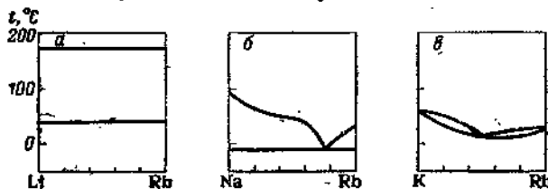
Рис. 2.46. Диаграммы состояния систем из некоторых щелочных металлов:
