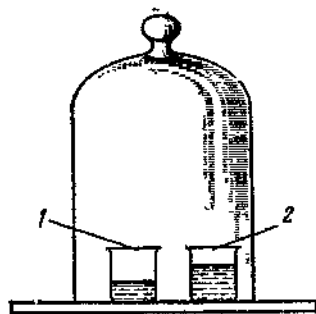
Рис. 2.25. Схема измерения давления насыщенного пара.
