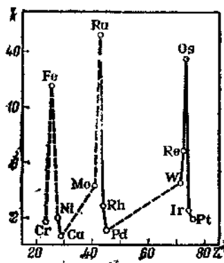
Рис. 2.18. Зависимость каталитической активности k некоторых элементов (для процесса разложения аммиака при 600 °C и 101 кПа) от их порядкового номера Z .
