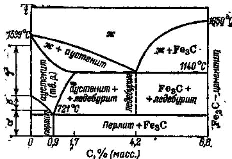
Рис. 3.124. Диаграмма состояния системы Fe—C (упрощенная).
