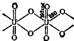
Рис. 3.152. Фрагмент структуры \text{MgUO}_4(\text{к}) .
