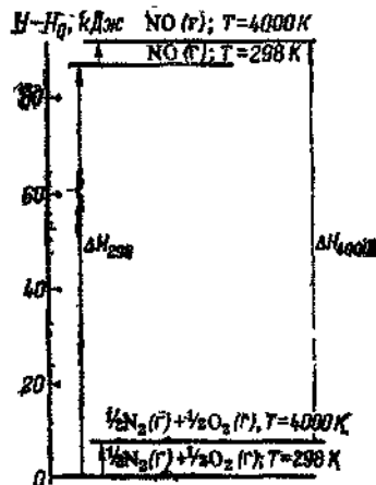
Рис. 2.2. Энтальпийная диаграмма для расчета влияния температуры на тепловой эффект реакции 1/2\text{N}_2(\text{г}) + 1/2\text{O}_2(\text{г}) = \text{NO}(\text{г})
