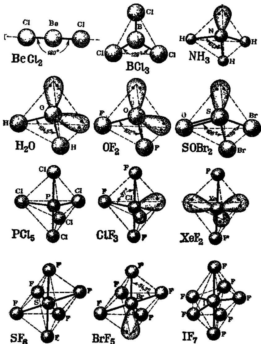
Рис. 1.27. Примеры для объяснения конфигурации различных молекул с помощью модели отталкивания электронных пар.
