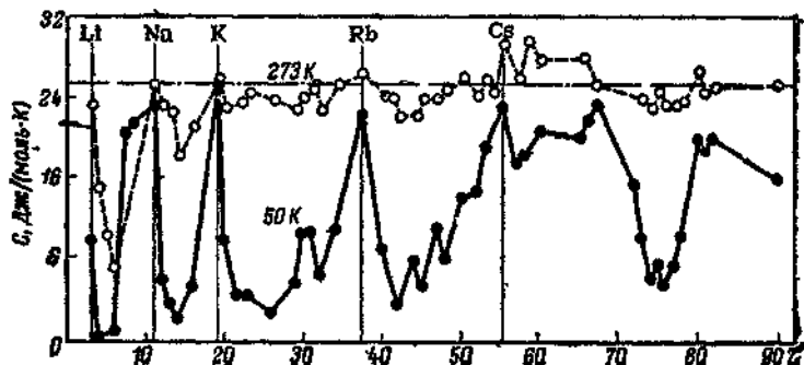
Рис. 113. Зависимость атомной теплоемкости от порядкового номера элемента.
