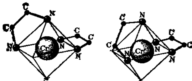
Рис. 1.58. Схематическое изображение структур зеркальных изомеров комплексов хрома с этилендиамином.
