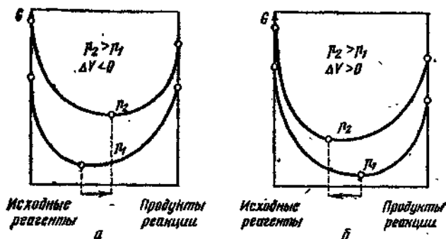
Рис. 2.13. Влияние давления на химическое равновесие при T = \text{const} : а — реакция, сопровождающаяся уменьшением объема; б — реакция, сопровождающаяся увеличением объема. По оси абсцисс отложен состав смеси.
