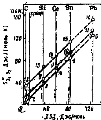
Рис. 3.32. Взаимосвязь между стандартными энтропиями изoeлектронных бинарных соединений S_1, S_2 и элементных веществ S подгруппы IVA:
