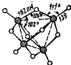
Рис. 3.55. Строение молекул P_4O_6 и P_4O_{10} .
