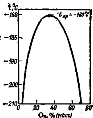
Рис. 3.64. Диаграмма растворимости в системе O_2-O_3 .
