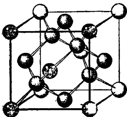
Рис. 1.85. Структура алмаза.
