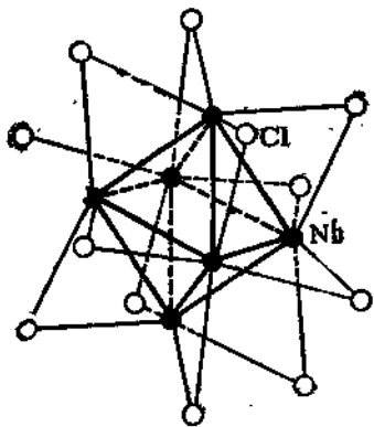
Рис. 3.94. Строение иона (\text{Nb}_6\text{Cl}_{12})^{2+} .
