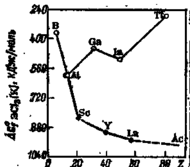
Рис. 2.98. Зависимость стандартных энтальпий образования хлоридов элементов III группы от порядкового номера элемента.
