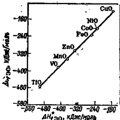
Рис. 3.97. Взаимосвязь между стандартными энтальпиями и энергиями Гиббса образования оксидов d-элементов четвертого периода.
