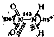
Рис. 3.61. Строение молекул нитрамида.
