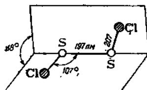
Рис. 3.70. Строение молекулы \text{S}_2\text{Cl}_2 .
