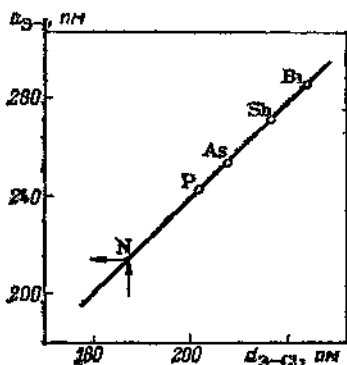
Рис. 1.16. Взаимосвязь межатомных расстояний \Theta - I и \Theta - Cl .
