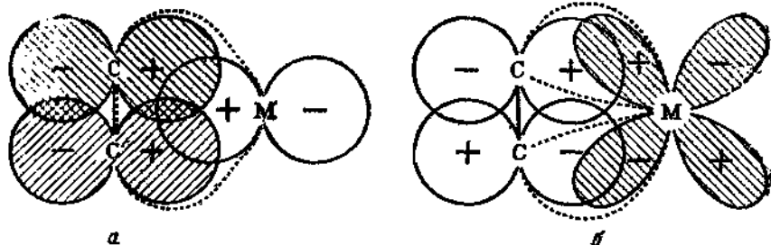
Рис. 1.68. Схемы, показывающие образование связей и \pi -комплекса с этиленом в качестве лиганда:
