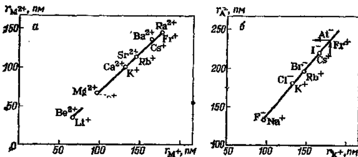
Рис. 1.19. Сопоставление радиусов ионов металлов IА и IIА подгрупп (а) и изoeлектронных ионов щелочных металлов и галогенов (б).
