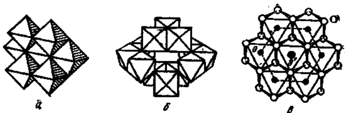
Рис. 3.115. Структура некоторых изо- и гетерополианионов, построенных из октаэдрических групп \text{MoO}_6 и \text{WO}_6 :
