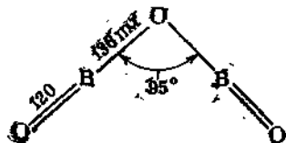
Рис. 3.9. Строение молекулы B_2O_3 .
