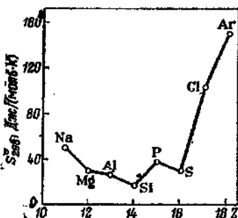
Рис. 2.6. Зависимость стандартной энтропии элементарных веществ третьего периода от порядкового номера элементов.
