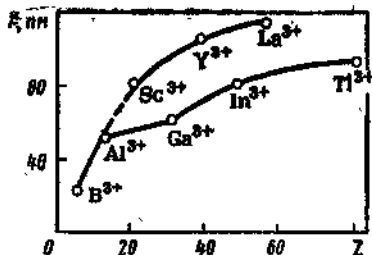
Рис. 3.14. Зависимость радиусов ионов элементов III группы от порядкового номера.
