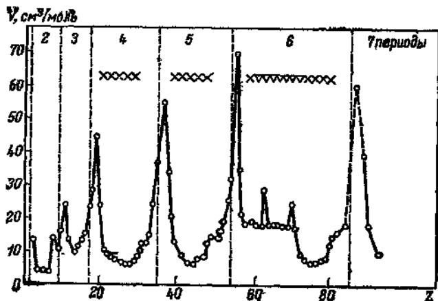
Рис. 1.11. Зависимость от порядкового номера элемента атомного объема простых веществ. Знаком X отмечены элементы побочных подгрупп, знаком V — лантаноиды.
