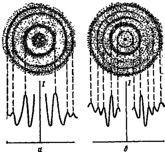
Рис. 1.25. Электрограммы \text{CCl}_4 (а) и \text{CS}_2 (б).
