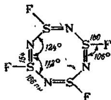
Рис. 3.73. Строение молекул \text{SF}_4 (а), (\text{NSF})_4 (б), (\text{NSF})_3 (в).
