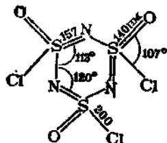
Рис. 3.75. Строение молекулы (NSOCl)_3 .
