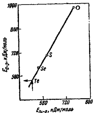
Рис. 1.22. Взаимосвязь энергий связи соединений кремния и углерода.
