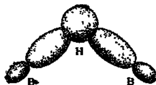
Рис. 1.56. Схема образования связей В—Н—В.
