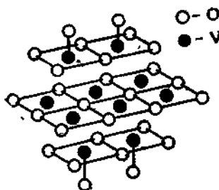
Рис. 3.109. Структура иона (\text{V}_{10}\text{O}_{28})^{4-} .
