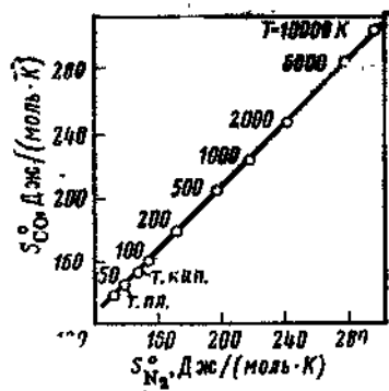
Рис. 3.25. Взаимосвязь между энтропиями N_2 и CO при одинаковых температурах.
