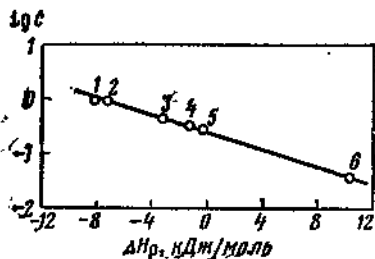
Рис. 2.19. Взаимосвязь между теплотой растворения \Delta H_p и растворимостью газов c в C_2H_5OH при 25^\circ C : 1 — He; 2 — Ne; 3 — N 2 ; 4 — CO; 5 — Ar; 6 — CO 2 .
