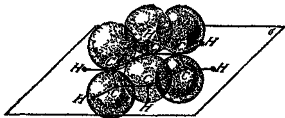
Рис 146 Схема, показывающая образование химических связей в молекуле C_6H_6 . Чтобы не загромождать чертеж, показаны только три p -орбитали.
