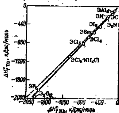
Рис. 3.104. Взаимосвязь между стандартными энтальпиями образования некоторых кристаллических соединений Nb и Ta.
