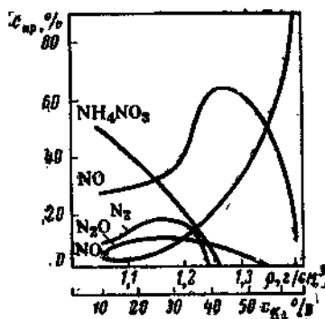
Рис 3.51. Зависимость содержания c_{\text{пр}} различных продуктов восстановления железом \text{HNO}_3 от ее плотности \rho (концентрации c_{\text{ж}} ).
