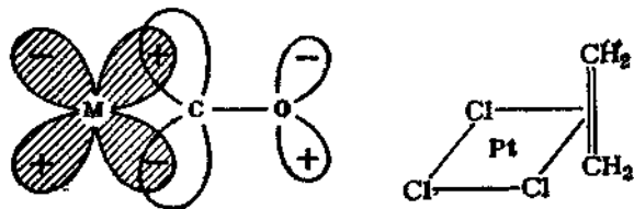
Рис. 1.66. Схема, показывающая образование \pi -связи между атомом металла и молекулой \text{CO} .
