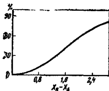
Рис. 1.57. Зависимость степени ионности связи P от разности электроотрицательностей элементов (по Полингу).
