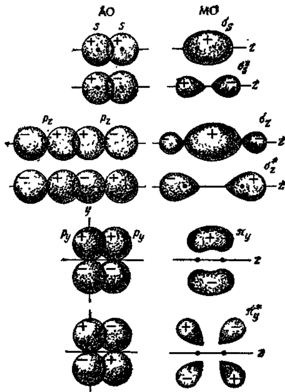
Рис. 1.50. Схема образования молекулярных орбиталей из атомных. + и - знаки волновой функции.
