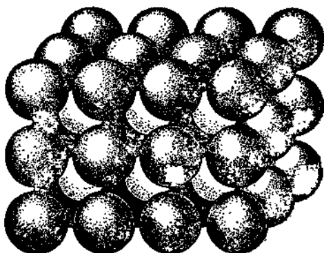
Рис. 1.83. Кристаллическая решетка хлорида цезия.
