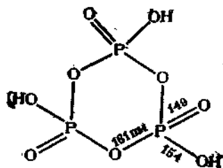
Рис. 3.59. Строение молекулы триметафосфорной кислоты.
