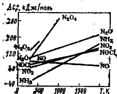
Рис. 3.50. Зависимость изменения стандартной энергии Гиббса образования некоторых соединений азота от температуры.
