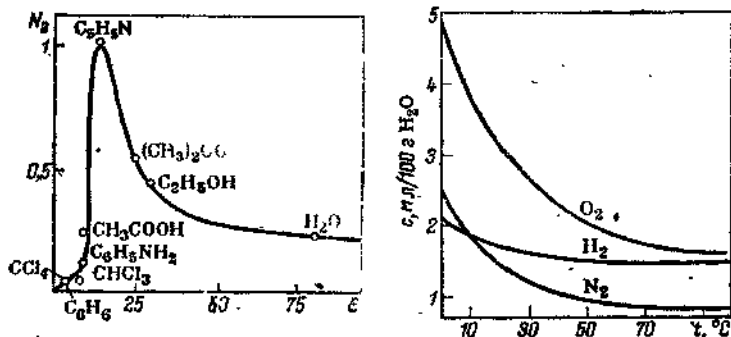
Рис. 2.20. Зависимость растворимости м-диоксибензола (резорцина) от диэлектрической проницаемости \epsilon растворителя при 30 °С. N_2 — мольная доля резорцина.
