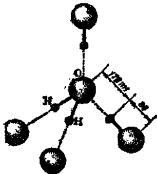
Рис. 1.7а. Фрагмент структуры льда.
