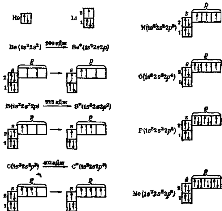
Рис. 1.34. Распределение электронов в атомах гелия и элементов второго периода по квантовым ячейкам.
