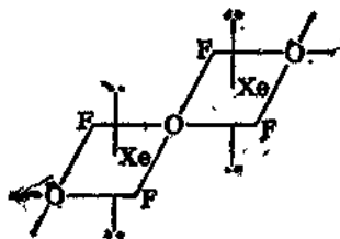
Рис. 3.89. Фрагмент структуры \text{XeOF}_2 (к).
