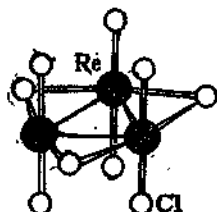
Рис. 3.120. Строение кластера Re_3Cl_9 .
