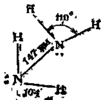
Рис. 3.47. Строение молекулы гидразина.
