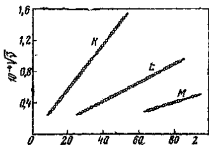
Рис. 144 Зависимость \sqrt{\nu} для линий серий K, L, M рентгеновского спектра от порядкового номера элемента.
