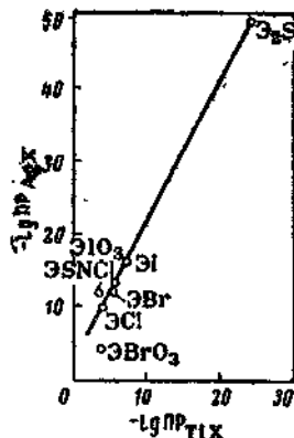
Рис. 3.15. Взаимосвязь между произведениями растворимости некоторых солей Tl^+ и Ag^+ при 25 °С
