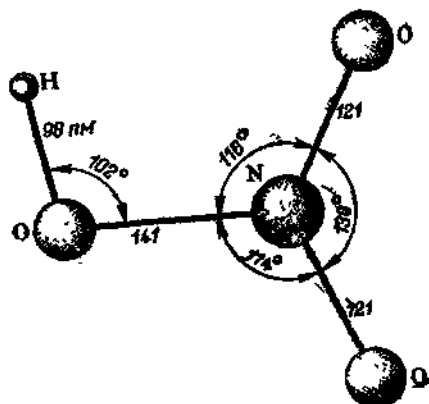
Рис. 1.48. Структура молекулы азотной кислоты.
