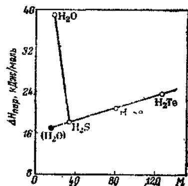
Рис. 1.89. Зависимость теплоты парообразования от молекулярной массы для водородных соединений VI группы.
