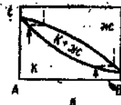
Рис. 331. Схема процесса зонной очистки (а) и диаграмма состояний системы с непрерывными рядами твёрдых растворов (б): I — перекристаллизованный материал; II — расплавленная зона; III — твёрдый (неиницированный) материал; 1 — фронт кристаллизации; 2 — фронт плавления.
