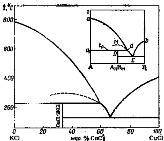
Рис. 2.37. Диаграмма состояния системы из веществ, образующих неустойчивое химическое соединение A_nB_m .
